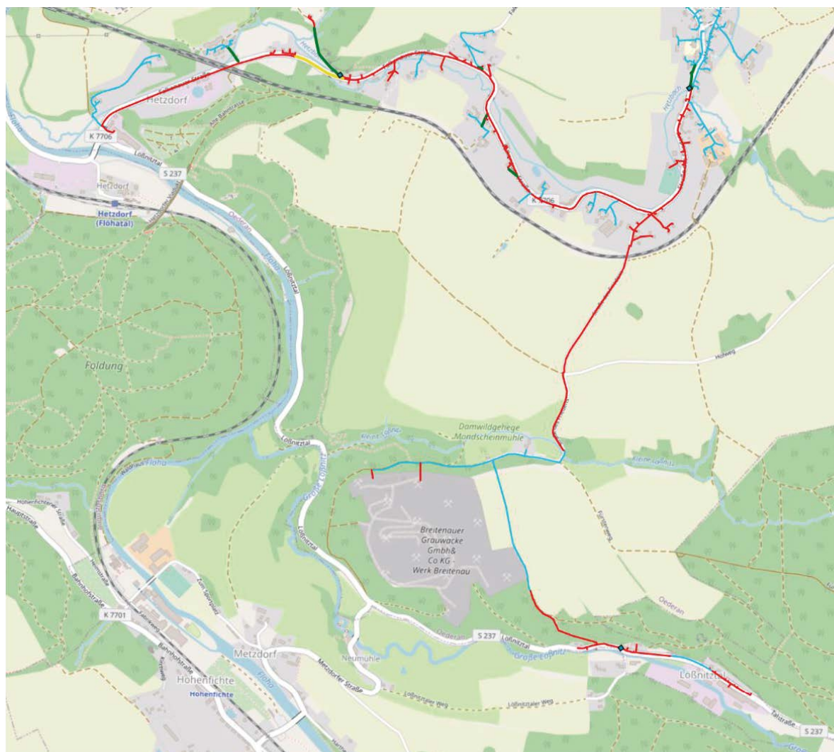
Bauumfang Stand 03/2023, Blau: Tiefbau fertig, Rot: wird jetzt ausgebaut
